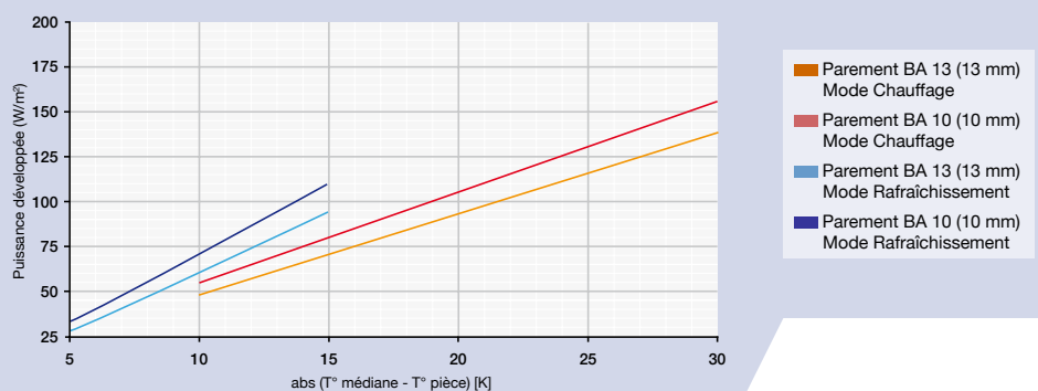
CD-4 - Performance en chauffage et rafraîchissement (Différence entre température moyenne de l'eau et température de la pièce)
